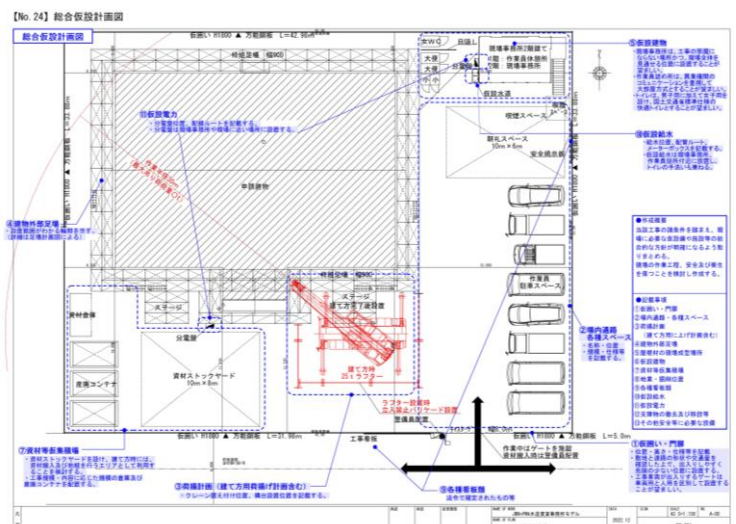
総合仮設計画図
